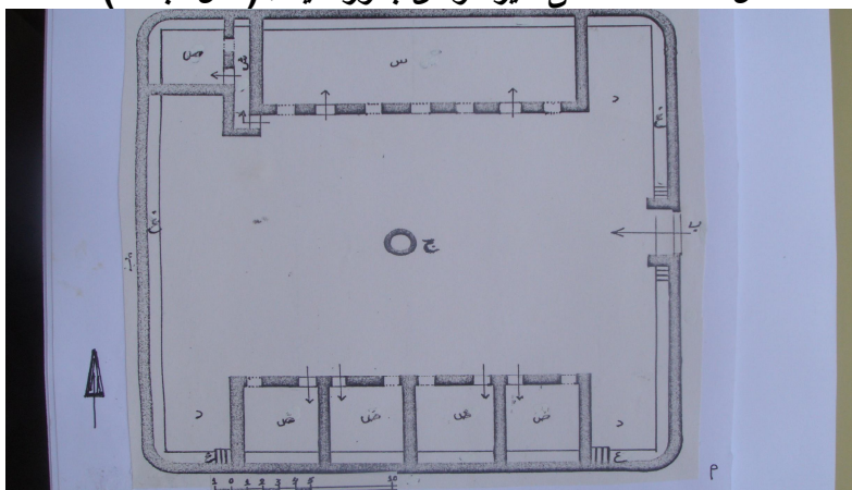
شكل ٣ - مسقط أفقي لقلعة نويبع - جنوب سيناء
