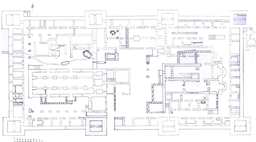
شكل ٢ - مسقط أفقي لدير الوادي بطور سيناء (عمل الباحث)
