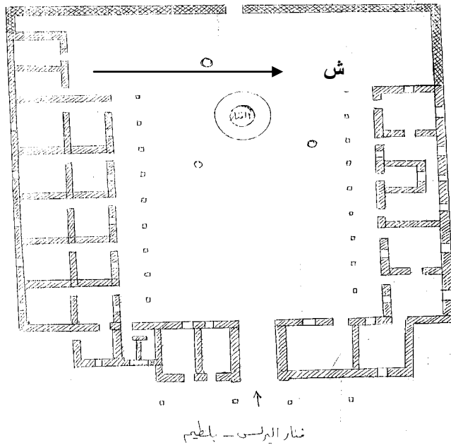
شكل (٣) المسقط الأفقي لفنار البرلس (عن المجلس الأعلى للآثار) شكل (٤) المسقط الأفقي لفنار المكس العالي (عن مصلحة الموانئ والمنائر)
