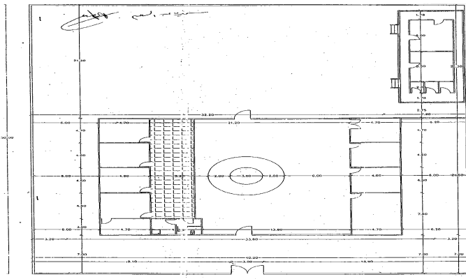
شكل (٣) المسقط الأفقي لفنار البرلس (عن المجلس الأعلى للآثار) شكل (٤) المسقط الأفقي لفنار المكس العالي (عن مصلحة الموانئ والمنائر)
