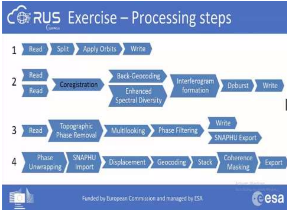
(شكل ٦) الخطوات التي تم القيام بها لتحليل صور الأقمار الصناعية الرادارية للحصول على قيم الهبوط الأرض
