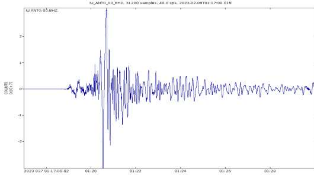
(شكل ٥) مخطط الزلازل هو مخرج رسم بياني بواسطة مخطط الزلازل. إنه سجل للحركة الأرضية في محطة القياس كدالة للزمن
