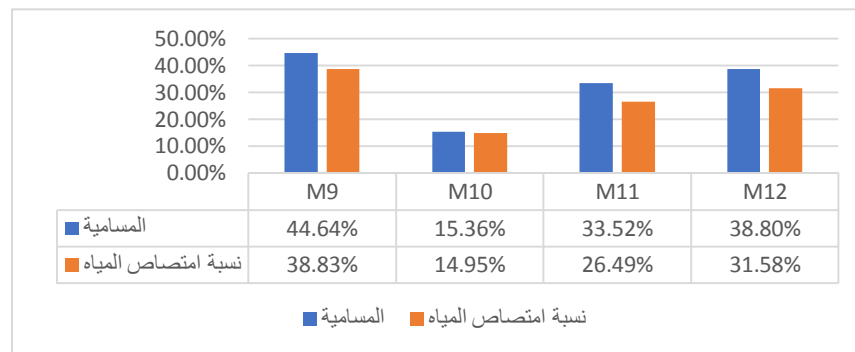
(شكل ٧) يوضح نسبة المسامية وامتصاص المياه للعينات التجريبية المضاف لها الرماد المتطاير ©عمل الباحثة
