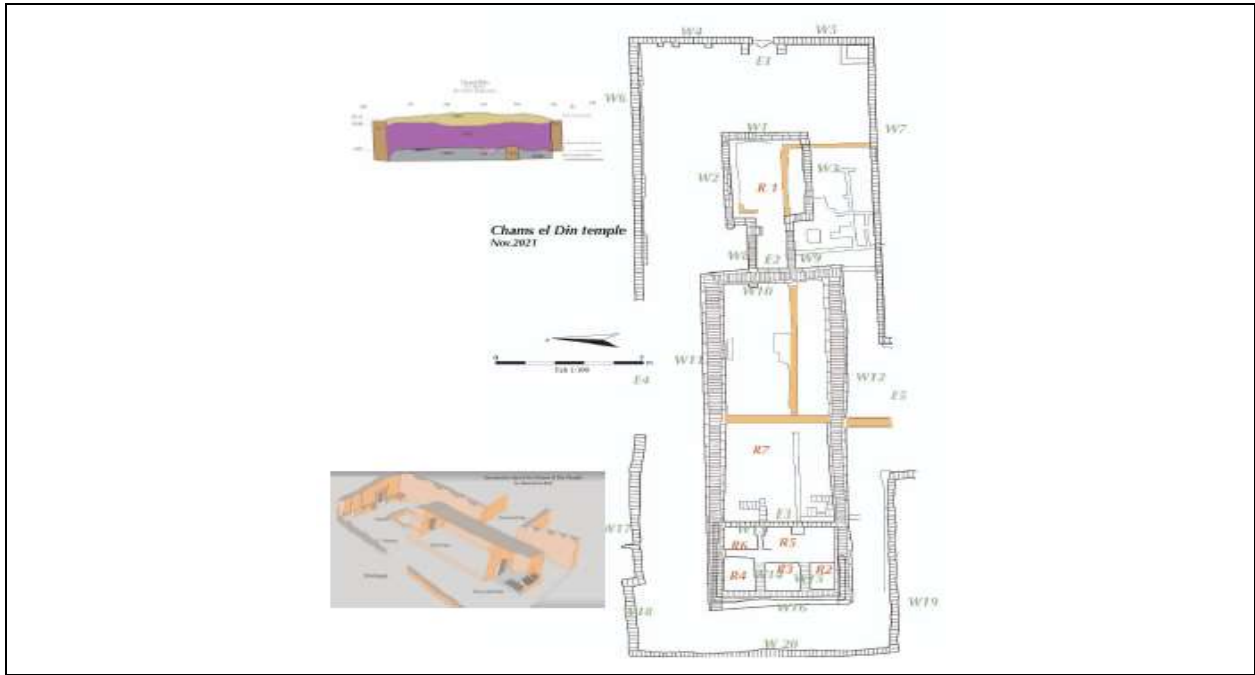
(شكل ٣) مسقط أفقي للمعبد الروماني بمنطقة شمس الدين ق ٣-٤م- عن: المجلس الأعلى للآثار، تقرير حفائر البعثة المصرية النرويجية المشتركة بواحة الخارجة، ٣٠.
